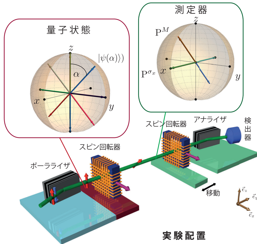
図2 実験配置図。実験用原子炉から取り出された中性子は、青の部分にあるポーライザで状態 \Psi に初期化される。次に、パラメータ掃引法を実行するために赤の部分にあるスピントルネーターで初期状態をパラメータ値 t だけ変化させて \Psi(t)=U(t)\Psi に変換する。緑の部分では、3状態法に必要な操作を行った後に、アナライザでスピントルネーター測定を行う。これらの測定によって得られたデータから、状態 \Psi(t) における量子二乗平均平方根誤差の値を計算する。
